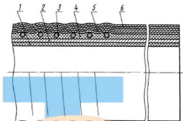
Схема конструкции рукава
